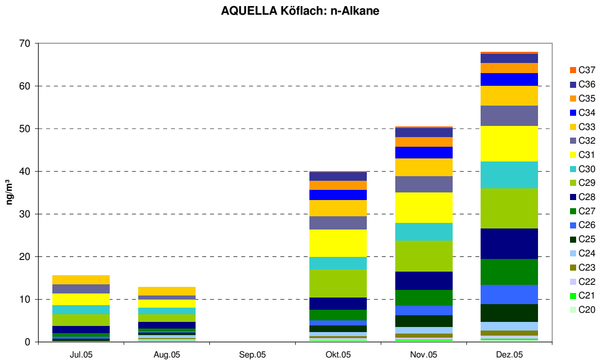
Abbildung 12: n-Alkane Monatsmittelwerte
