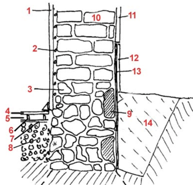
Vertikalabdichtung, Quelle: NÖ-Gestaltungsakademie
