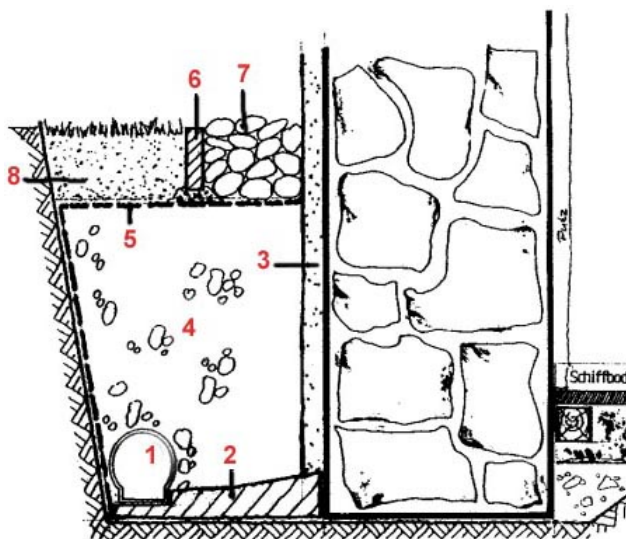
Fachgerechte Drainage, Quelle: Bohinc GmbH
