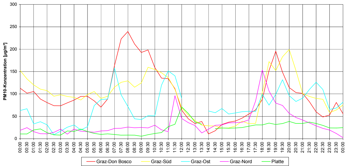
PM10-Konzentrationen (HMW) am 17.03.2004 an den Grazer Luftgütemessstellen
