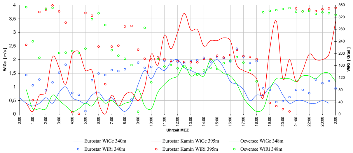
Windverhältnisse am 17.03.2004 an den Stationen Eurostar, Eurostar Kamin und Oeversee
