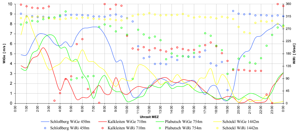
Windverhältnisse am 17.03.2004 an den Stationen Schloßberg, Kalkleiten, Plabutsch und Schöckl
