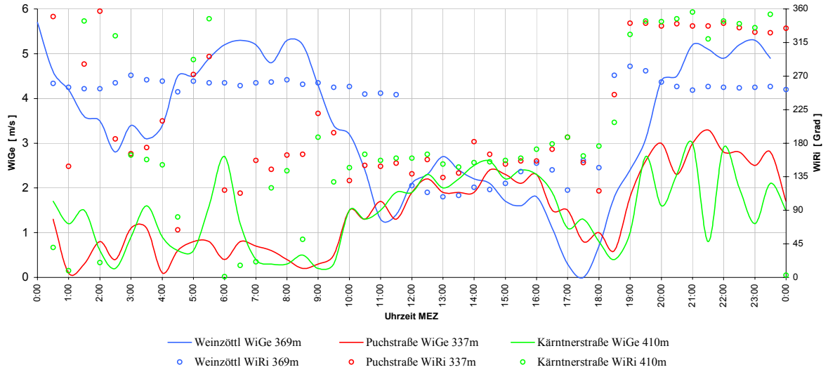
Windverhältnisse am 17.03.2004 an den Stationen Weinzöttl, Puchstraße und Kärntnerstraße
