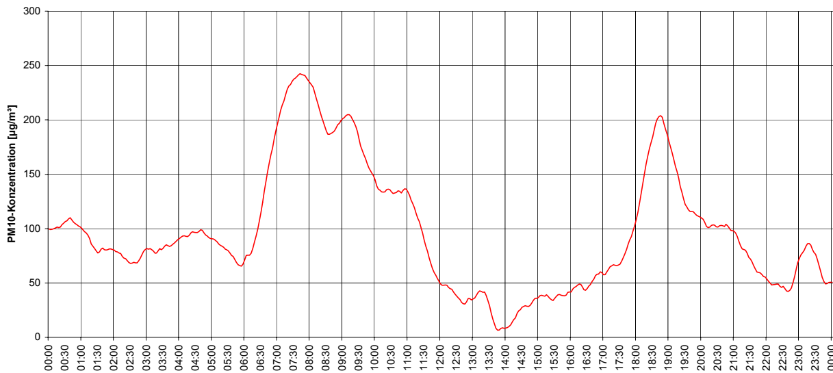
PM10-Konzentrationen (3-Minutenmittel) am 17.03.2004 an der Grazer Luftgütemessstelle Don Bosco
