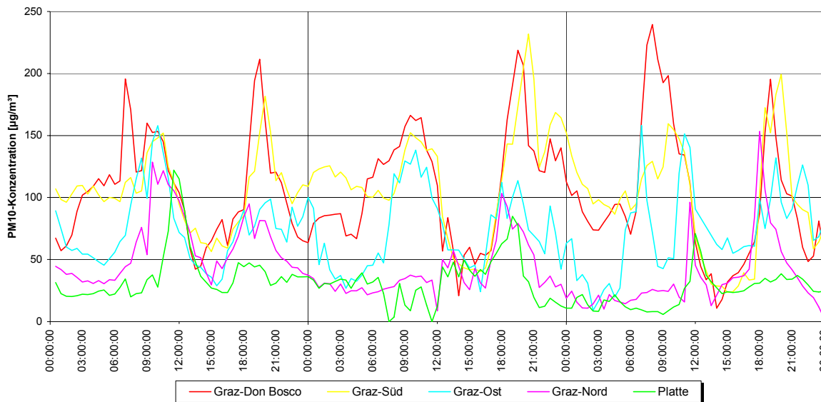
PM10-Konzentrationen (HMW) vom 15.-17.3.2004 an den Grazer Luftgütemessstellen
