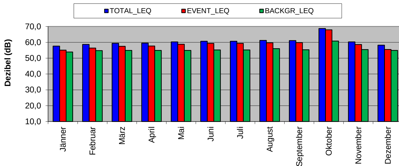
Messstation NMT 1 Graz-Süd: Jänner bis Dezember 2010
