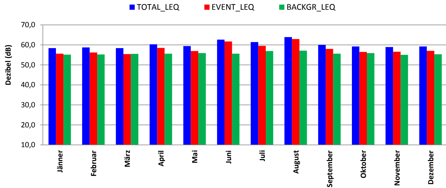
Messtation NMT 1 Graz-Süd: Jänner bis Dezember 2011
