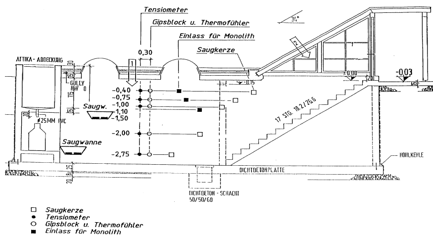
Abbildung 2: Längsschnitt durch die Lysimeteranlage in Wagna mit den Einlässen für die unterschiedlichen Messsonden und Probenahmesysteme
