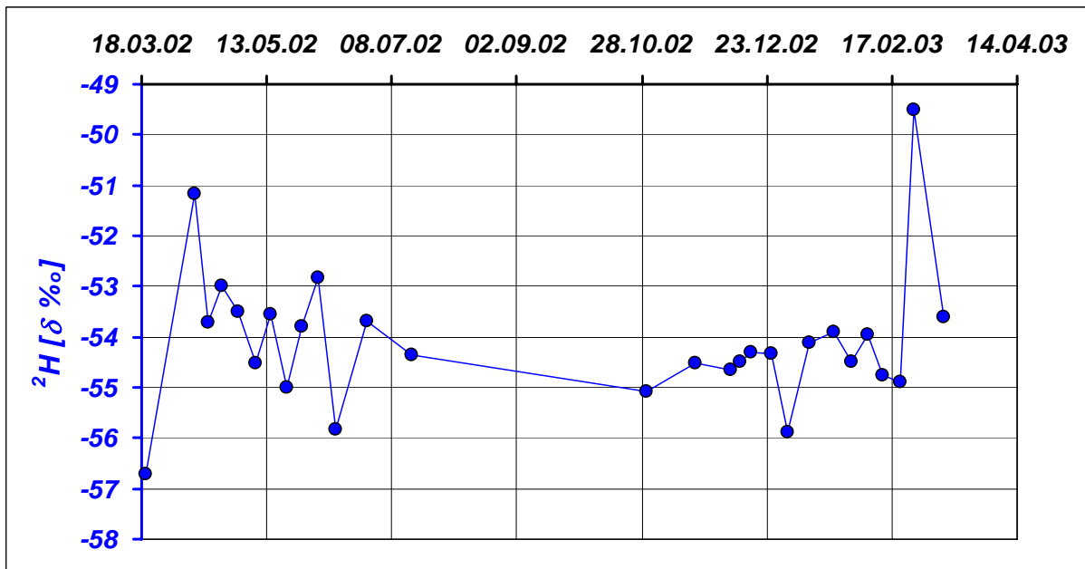
Abbildung 25: Deuterium-Analyseergebnisse an der Messstelle LSWL15 (Sickerwassersammler, FF, -1,50 m)
