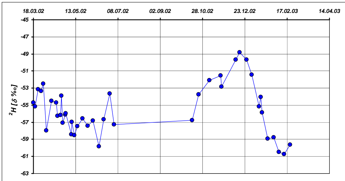
Abbildung 31: Deuterium -Analysenergebnisse an der Messstelle LSWR15 (Sickerwassersammler, MM,-1,50m)
