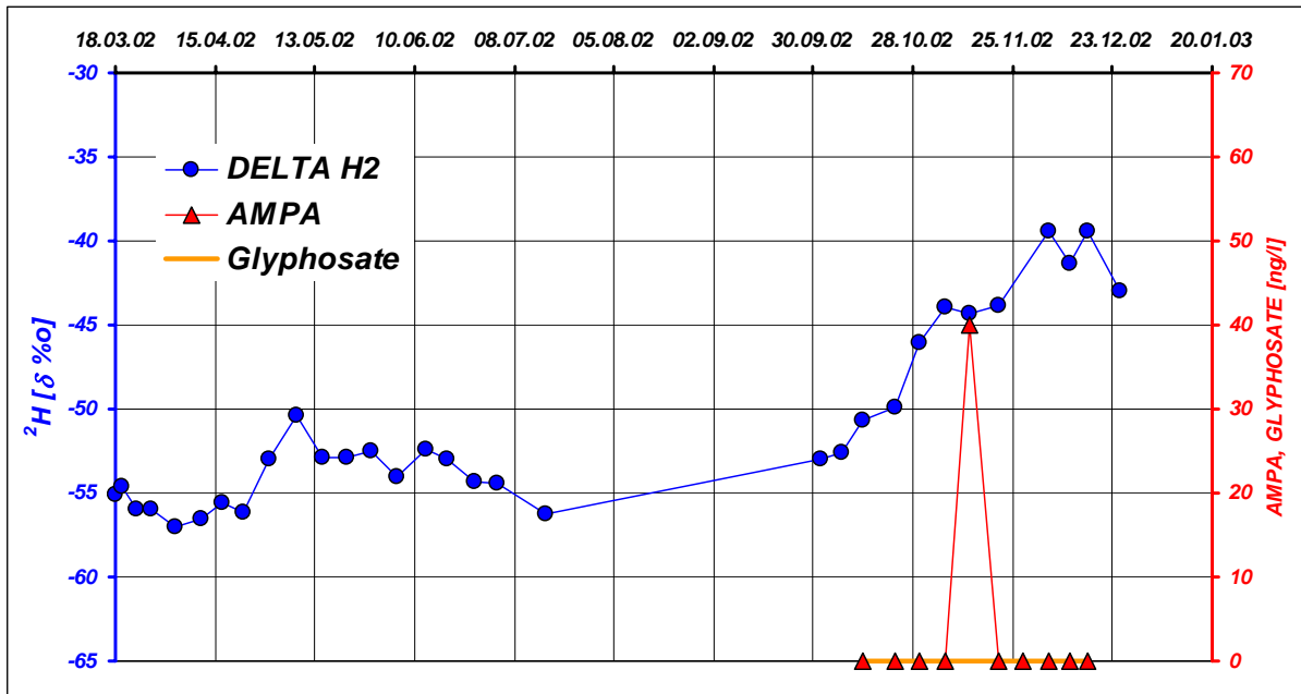
Abbildung 18: Deuterium-, Glyphosate- und AMPA-Analysenergebnisse an der Messstelle B6 (Saugkerze, FF,-1,05m)
