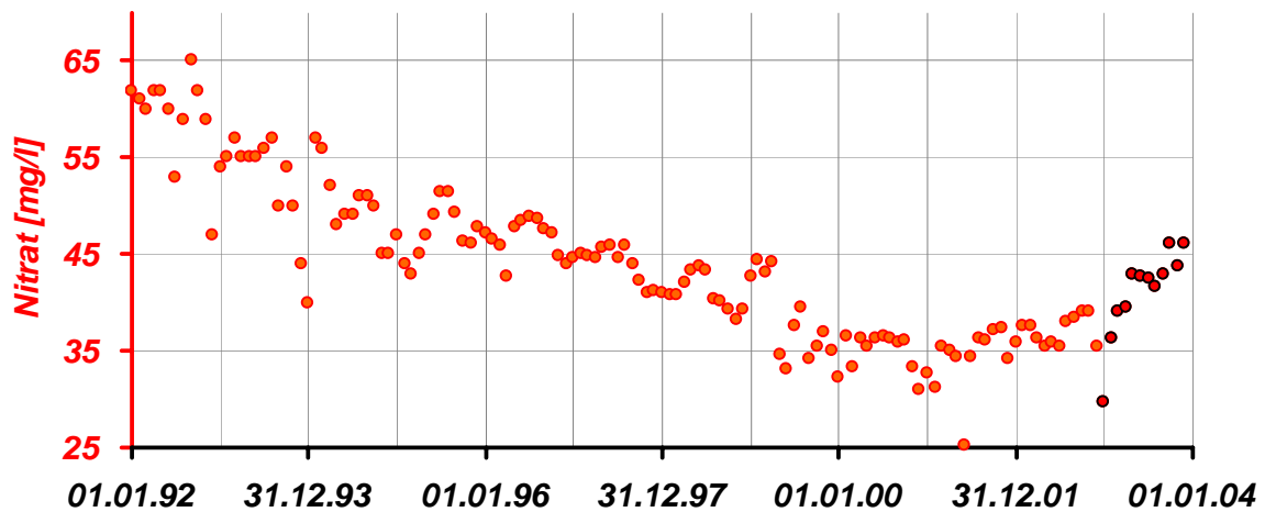
Abbildung 9: Entwicklung der Nitratkonzentration im Grundwasser des Jahres 2003 im Vergleich zum Beobachtungszeitraum 1992 – 2003
