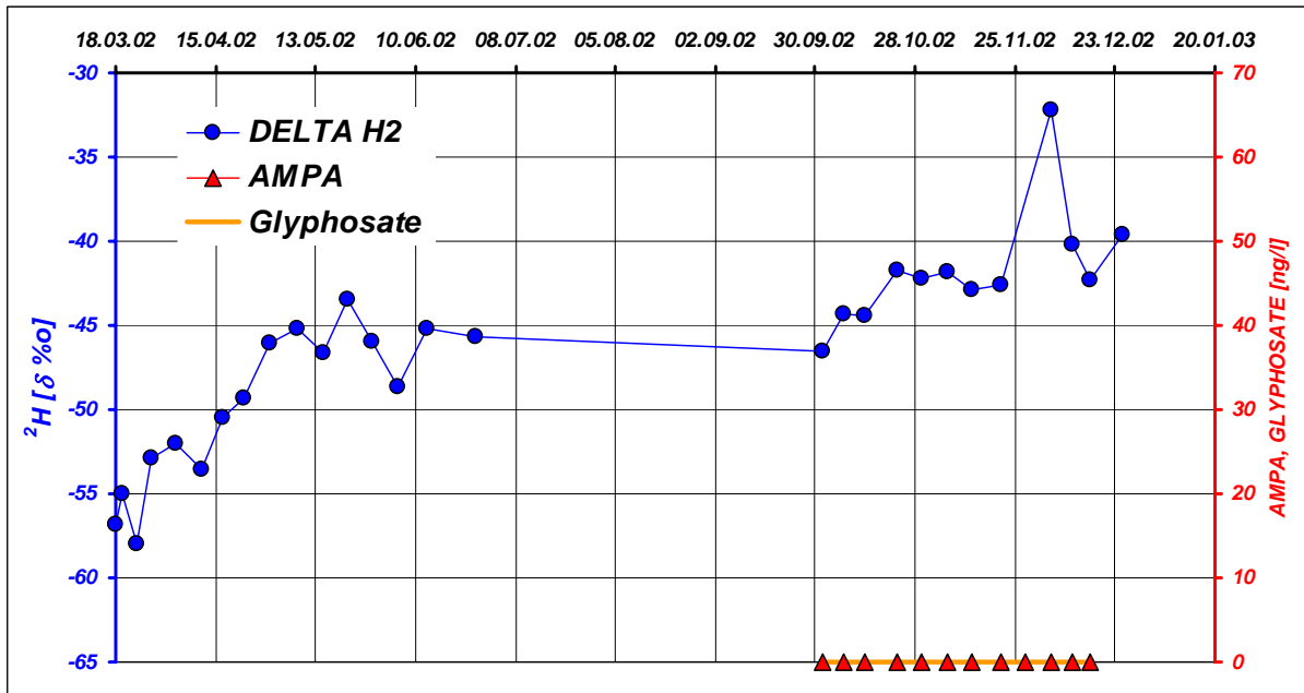
Abbildung 12: Deuterium-, Glyphosate- und AMPA-Analysenergebnisse an der Messstelle A5 (Sickerwassersammler, FF,-1,05m)
