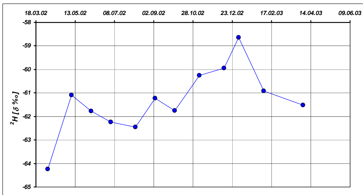
Abbildung 34: Deuterium -Analyseergebnisse an der Messstelle Grundwasser (Sonde)
