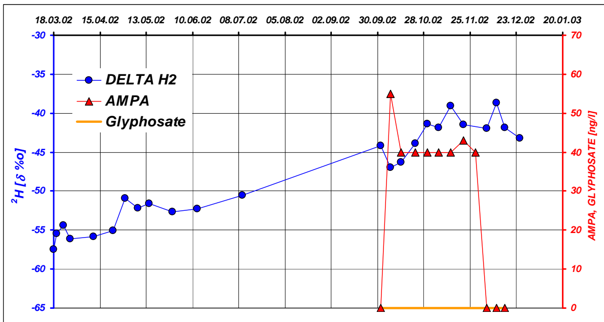
Abbildung 17: Deuterium-, Glyphosate- und AMPA-Analysenergebnisse an der Messstelle B4 (Sickerwassersammler, MM,-0,80m)
