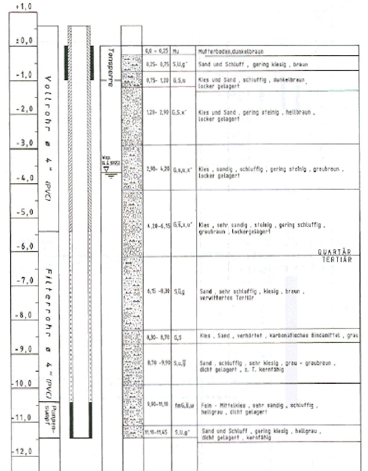
Abbildung 4: Bohrprofil und Ausbau der Bohrung Wagna II
