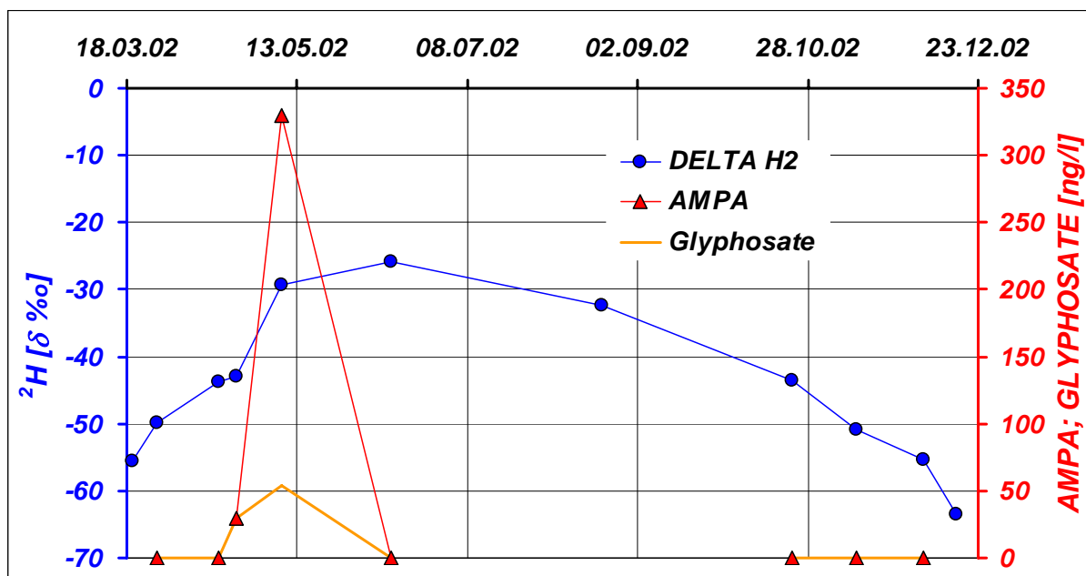
Abbildung 28: Deuterium-, Glyphosate- und AMPA-Analysenergebnisse an der Messstelle LSMR04 (Saugkerze, MM, -0,40m)
