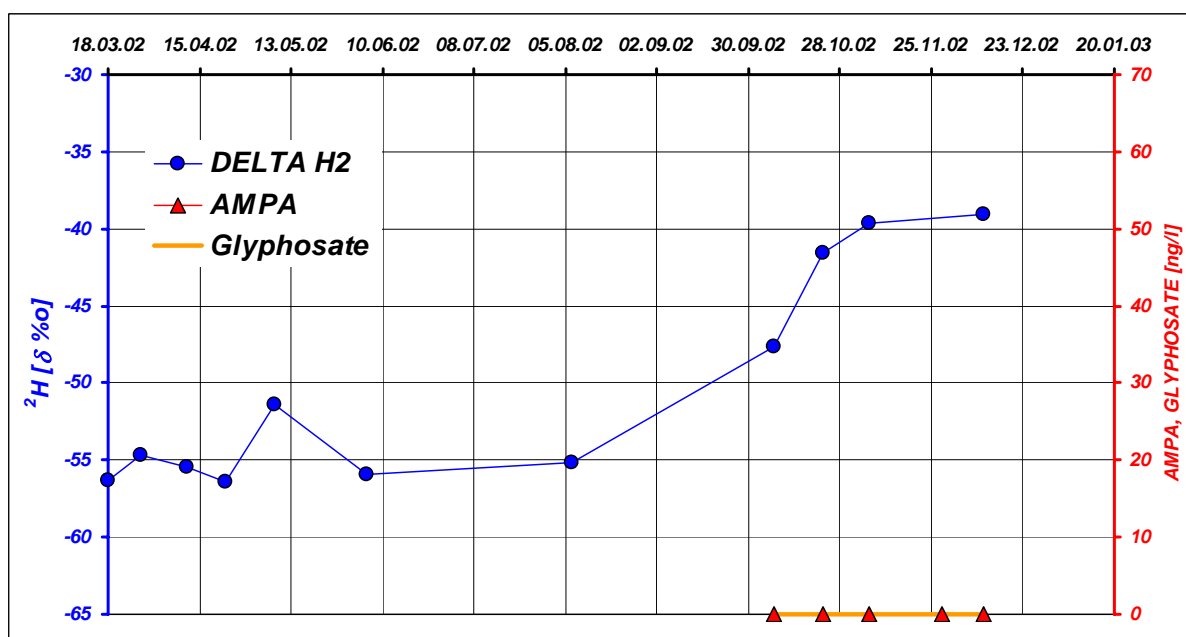
Abbildung 11: Deuterium-, Glyphosate- und AMPA-Analysenergebnisse an der Messstelle A4 (Saugkerze, MM,-0,80m)
