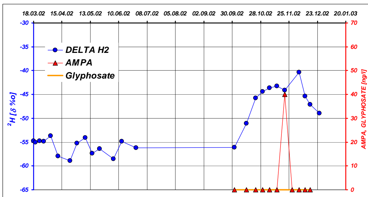
Abbildung 15: Deuterium-, Glyphosate- und AMPA-Analyseergebnisse an der Messstelle A8 (Saugkerze, FF, -1,05m)
