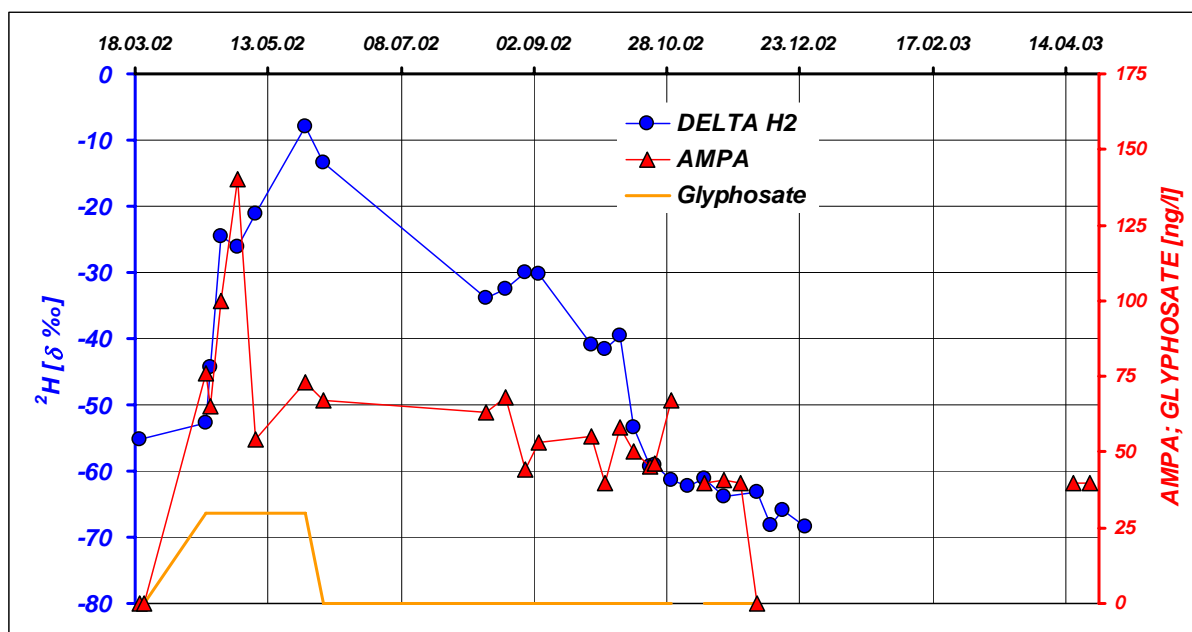
Abbildung 22: Deuterium-, Glyphosate- und AMPA-Analysenergebnisse an der Messstelle LSML04 (Monolithysimeter, FF,-0,40m)
