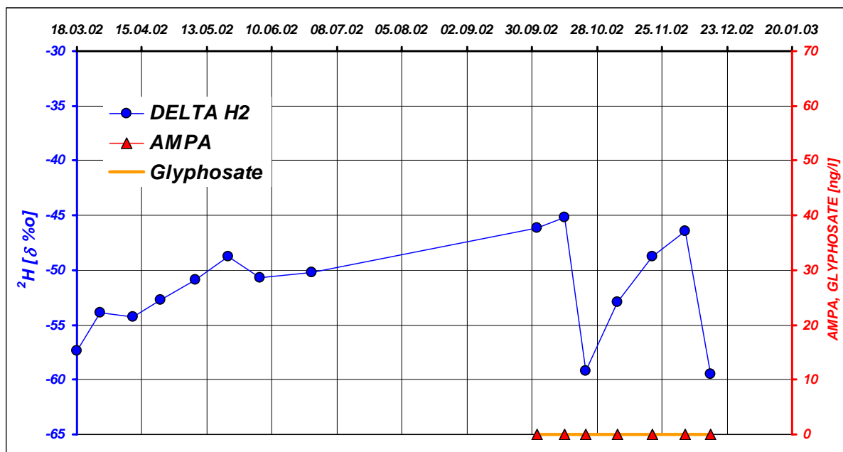
Abbildung 10: Deuterium-, Glyphosate- und AMPA-Analysenergebnisse an der Messstelle A1 (Saugkerze, MM,-0,80m)
