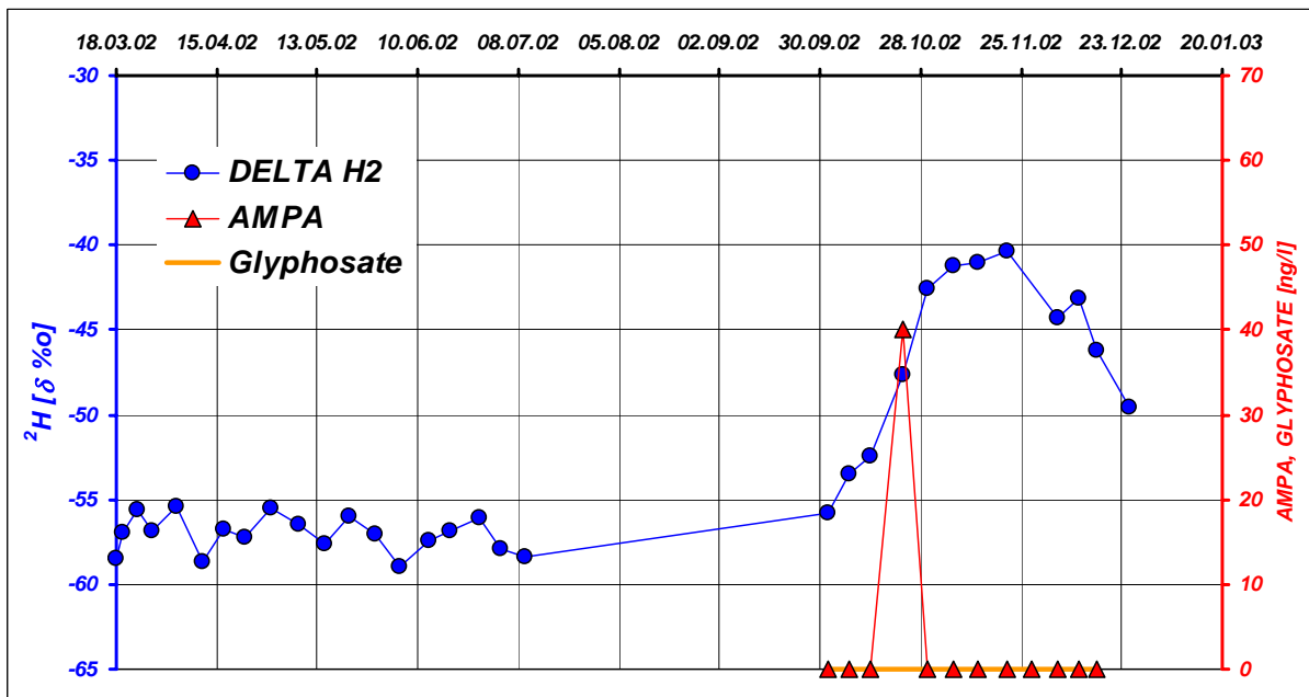
Abbildung 13: Deuterium-, Glyphosate- und AMPA-Analysenergebnisse an der Messstelle A6 (Saugkerze, FF,-1,05m)
