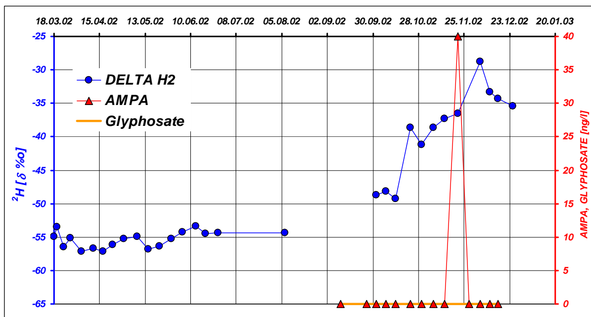
Abbildung 14: Deuterium-, Glyphosate- und AMPA-Analyseergebnisse an der Messstelle A7 (Saugkerze, MM, -0,80m)
