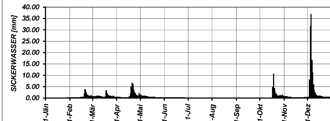
Jahresganglinie Messstelle WAGNA_SIWA_LSGVL 2002
