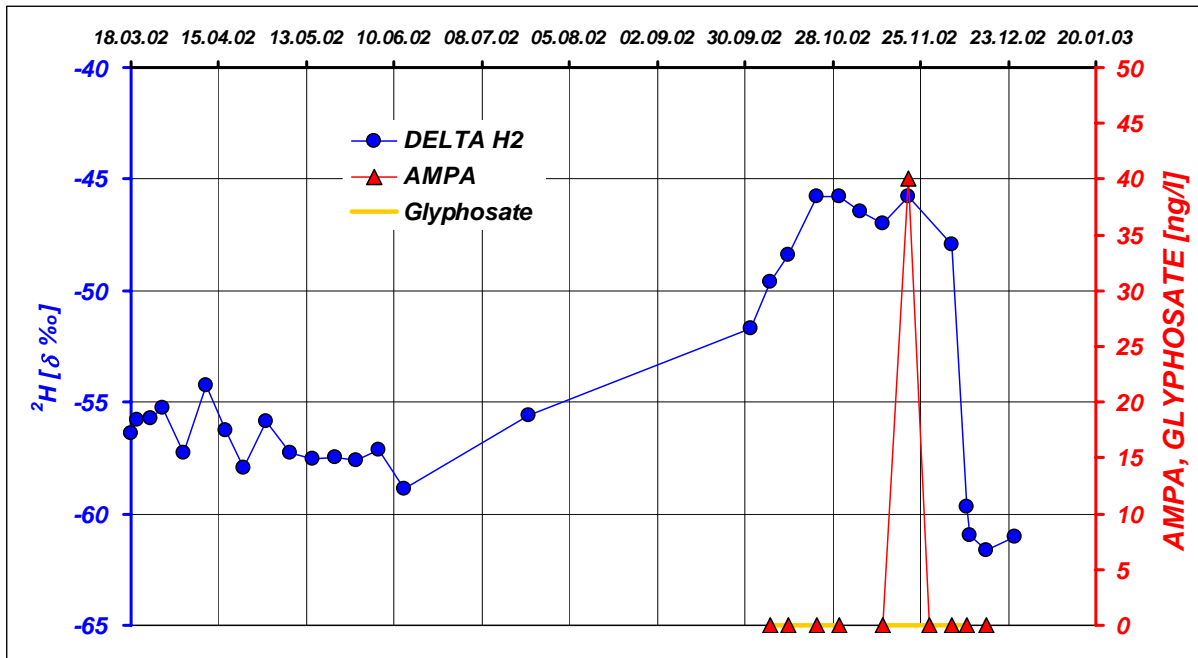
Abbildung 30: Deuterium-, Glyphosate- und AMPA-Analysenergebnisse an der Messstelle LSMR07 (Monolithysimeter, MM,-0,70m)
