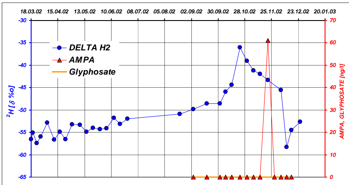
Abbildung 19: Deuterium-, Glyphosate- und AMPA-Analysenergebnisse an der Messstelle B7 (Saugkerze, MM,-0,80m)
