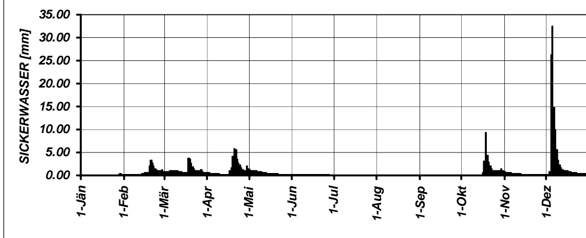
Jahresganglinie Messstelle WAGNA_SIWA_LSGVR 2002
