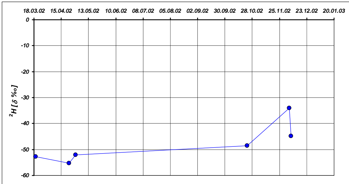
Abbildung 24: Deuterium -Analyseergebnisse an der Messstelle LSML11_A (Monolithysimeter, FF,-1,10m)
