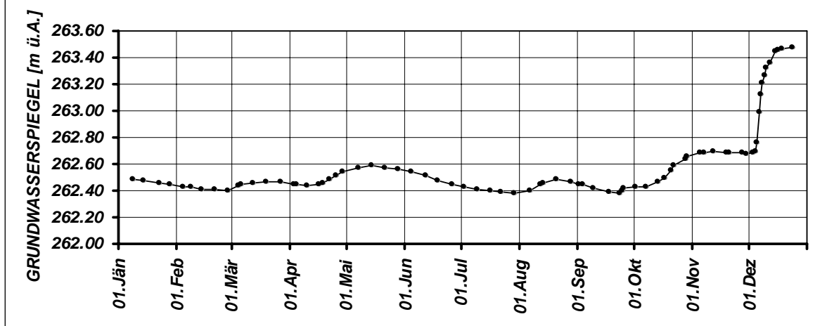
Jahresganglinie Messstelle WAGNA_GW_GWST_B1 2002
