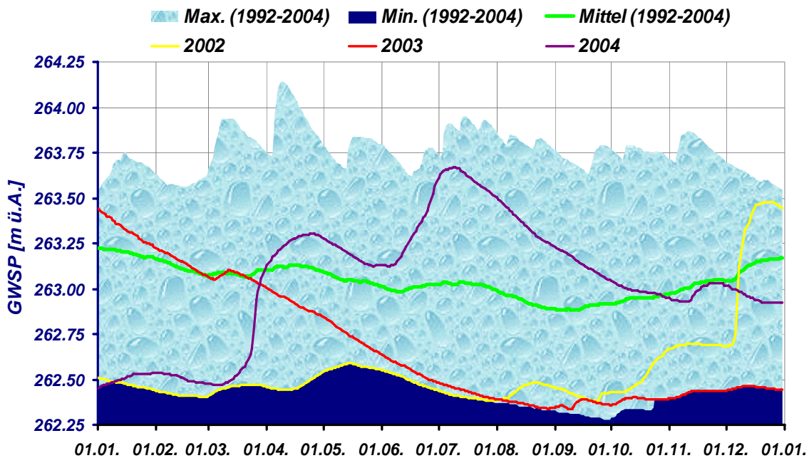
Abbildung 8: Grundwasserstandsganglinie 2003 im Vergleich zur mittleren Jahresgrundwasserstandsganglinie des Zeitraumes 1992 – 2004 und den in diesem Zeitraum auftretenden Minima und Maxima.
