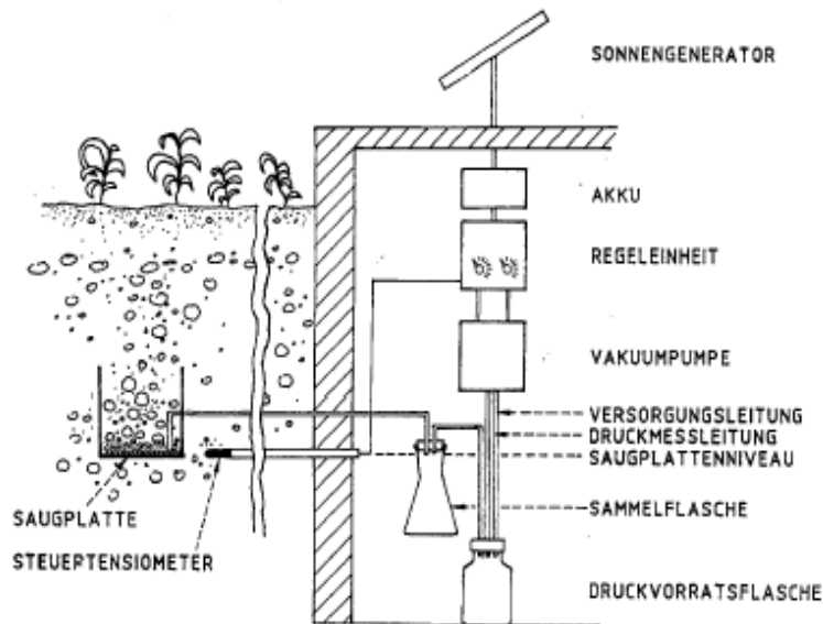
Abbildung 3: Schematische Darstellung des tensionsgesteuerten Unterdrucklysimeters
