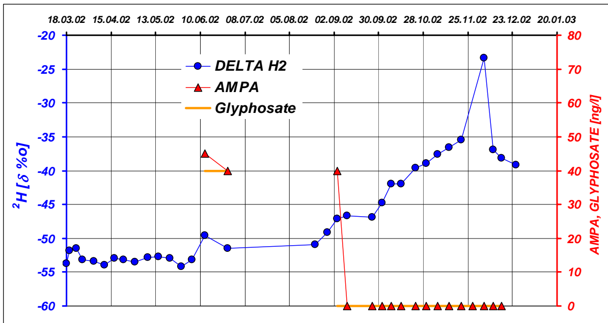
Abbildung 16: Deuterium-, Glyphosate- und AMPA-Analysenergebnisse an der Messstelle B1 (Sickerwassersammler, MM,-0,80m)
