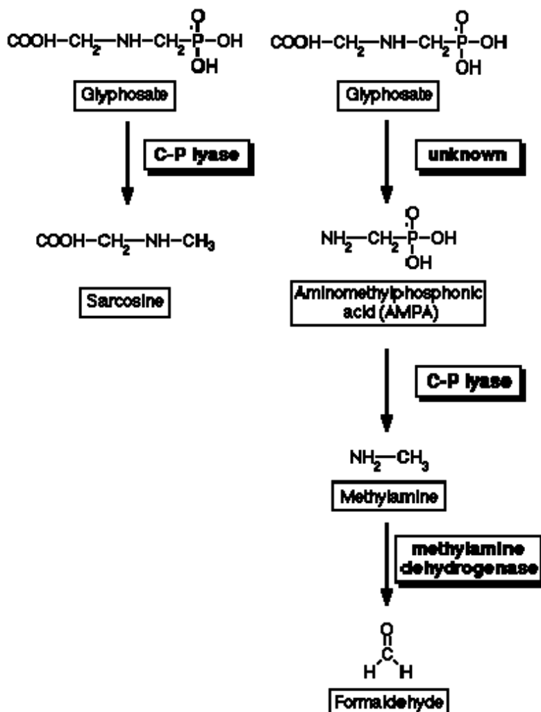
Abbildung 1: Abbauewege von Glyphosate
