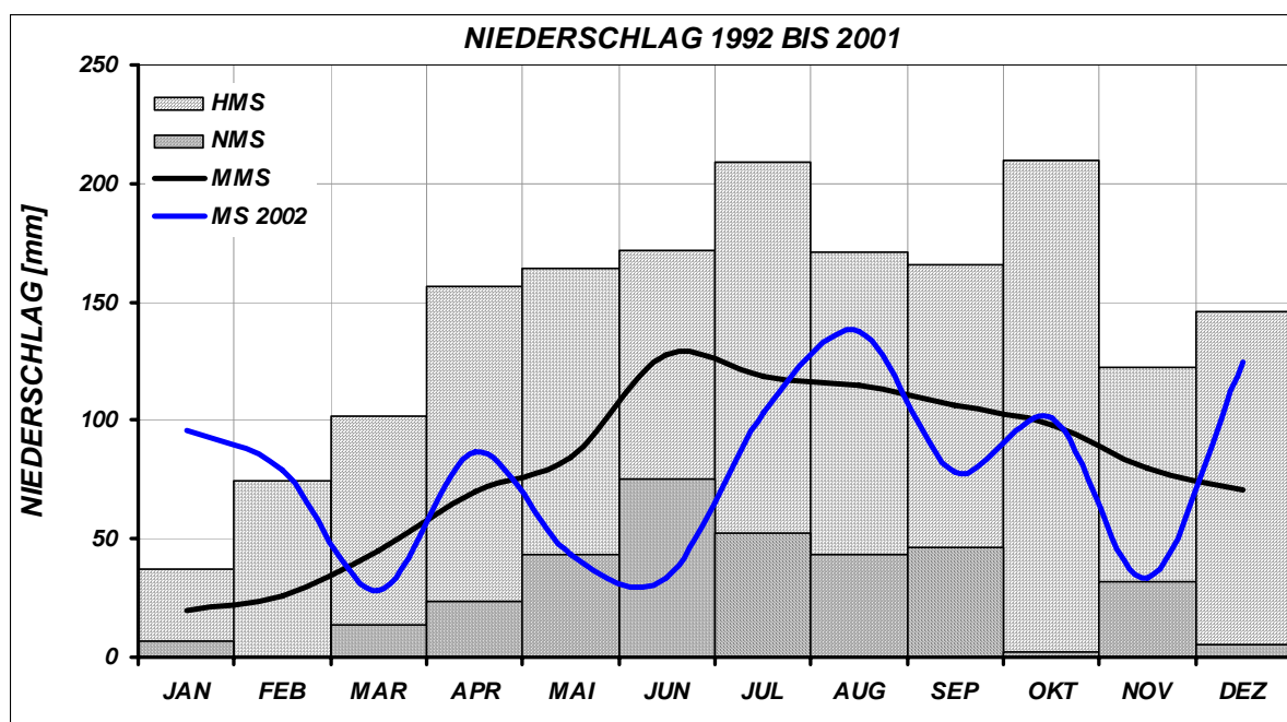
Abbildung 5: Monatssummen des Niederschlags des Jahres 2002 im Vergleich zu den niedersten (NMS), mittleren (MMS) und höchsten (HMS) Monatssummen der Reihe 1992 bis 2001.
