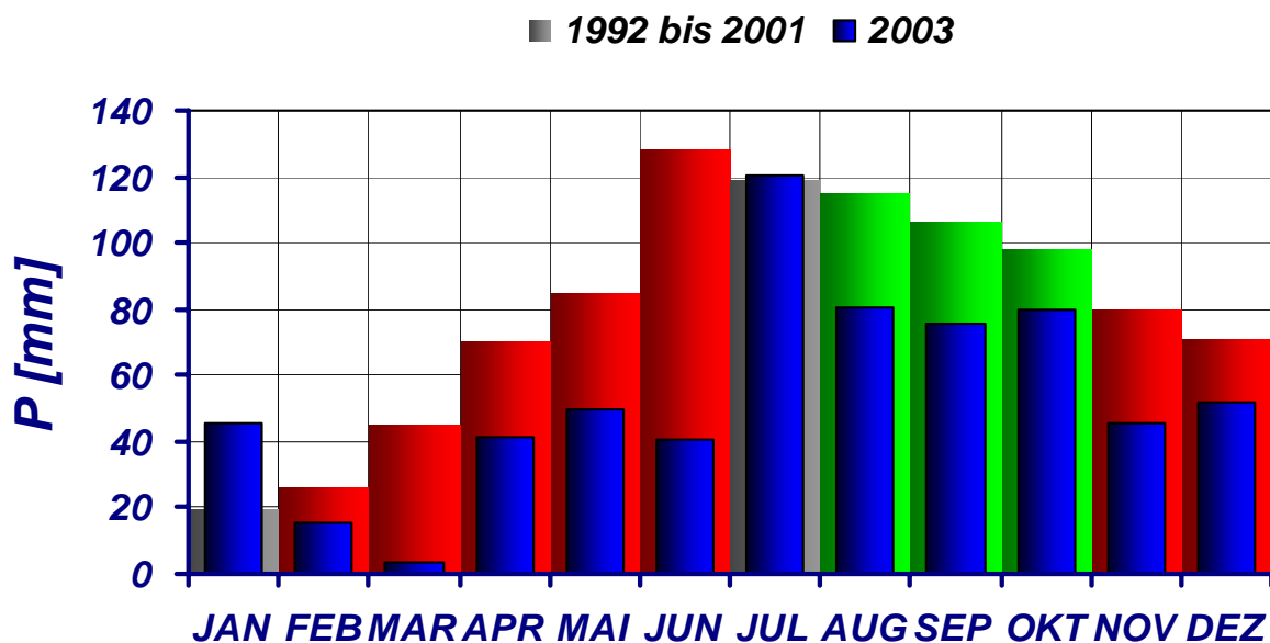
Abbildung 6: Niederschlagsverteilung des Jahres 2003 im Vergleich zur Reihe 1992 bis 2001
