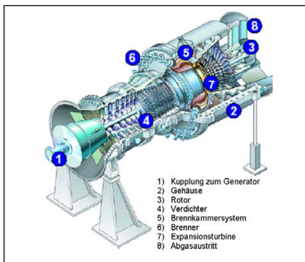
Abbildung 3-2: Schnitt durch eine Siemens V94.3A Gasturbine
