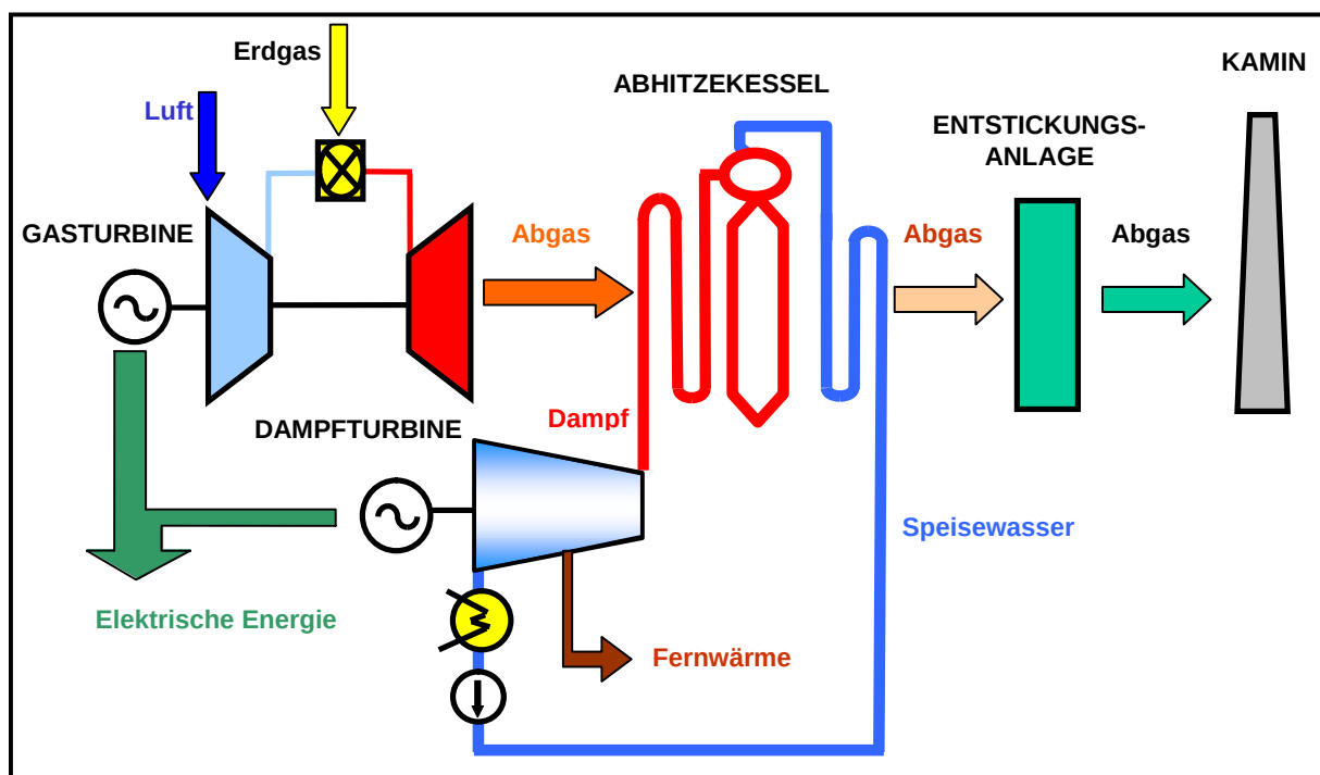
Abbildung 3-3: Vereinfachte Darstellung der Verstromungsschritte des GDK Mellach
