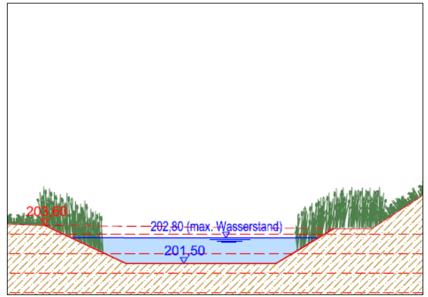
Abbildung 25: Schematische Profilskizze eines Himmelteichs
